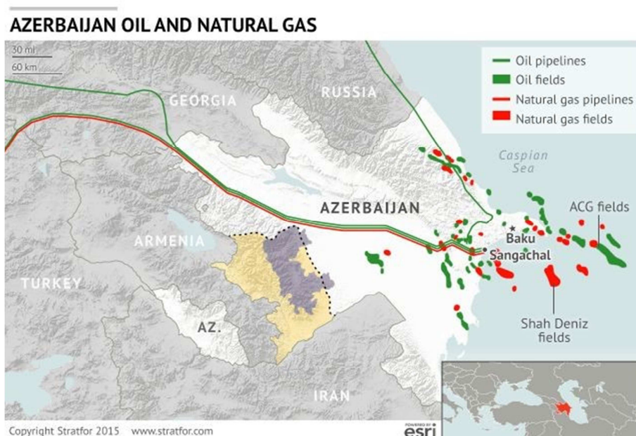
Εικόνα 3.2.3: Χάρτης των κοιτασμάτων υδρογονανθράκων και των υποδομών μεταφοράς πετρελαίου και φυσικού αερίου του Αζερμπαϊτζάν.
