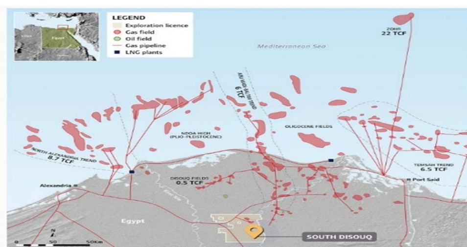
Εικόνα 3.2.4: Χάρτης των κοιτασμάτων φυσικού αερίου της Αιγύπτου πλησίον του Δέλτα του Νείλου.
