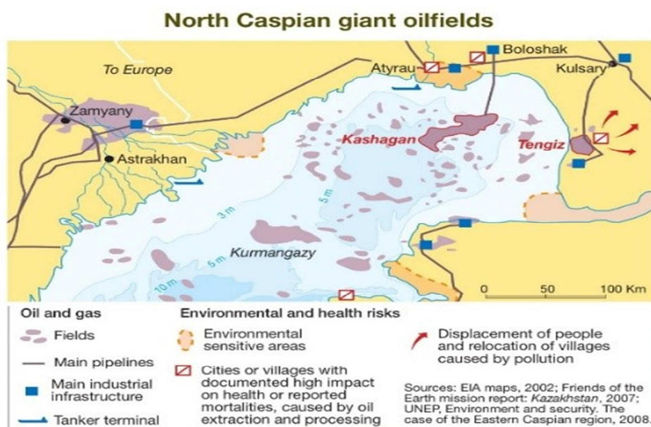
Εικόνα 3.2.2: Χάρτης των κοιτασμάτων υδρογονανθράκων του Καζακστάν στην Βόρεια Κασπία Θάλασσα. Διακρίνονται τα δύο μεγαλύτερα κοιτάσματα, το Τενγκίζ και το Κασάνγκαν.
